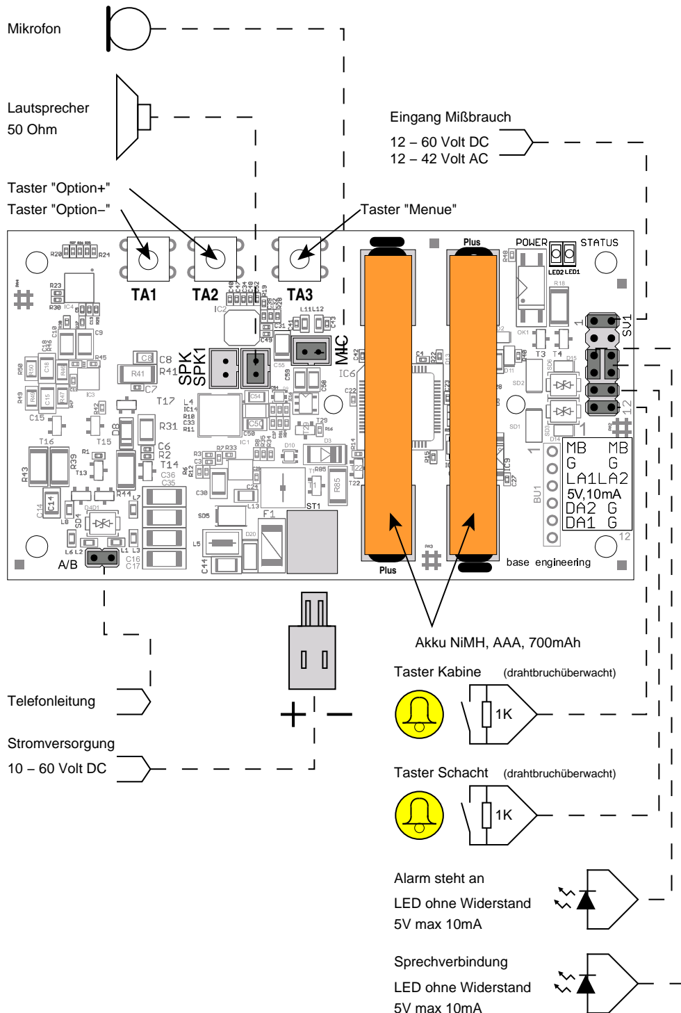
Abbildung 1: Anschlüsse des FWG12
