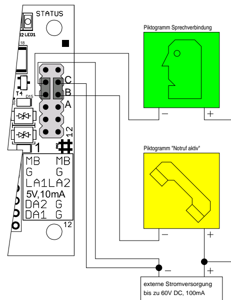
Piktogramme aus externer Stromversorgung versorgt
