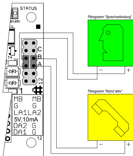
Piktogramme aus FGW12 versorgt, 5V, 10mA
